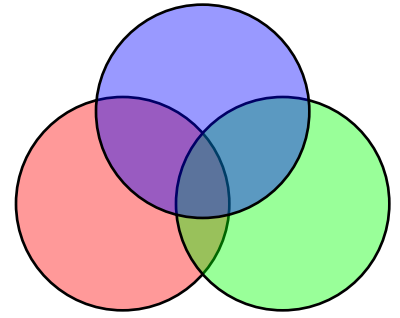
HPDF_BM_NORMAL alpha=0,4
